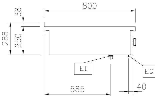
Zij aanzicht
