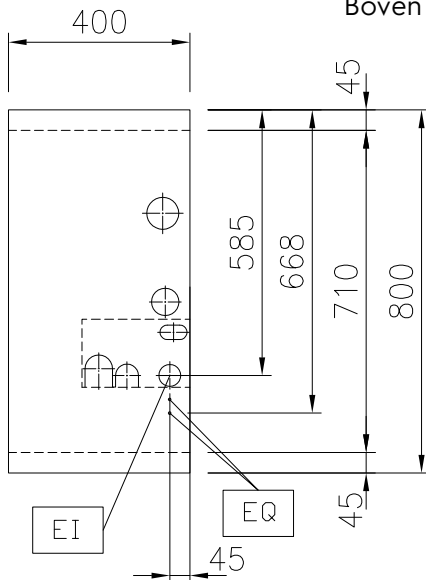
Boven aanzicht
